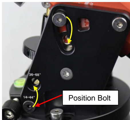
Figure 15. Change latitude range
